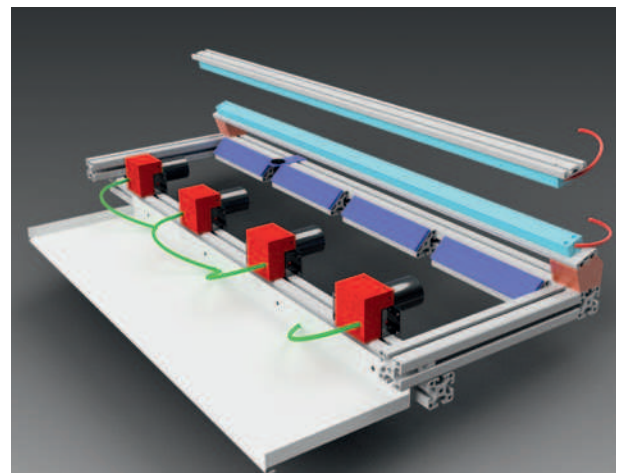
Kamerabaugruppe mit LED-Leuchten
