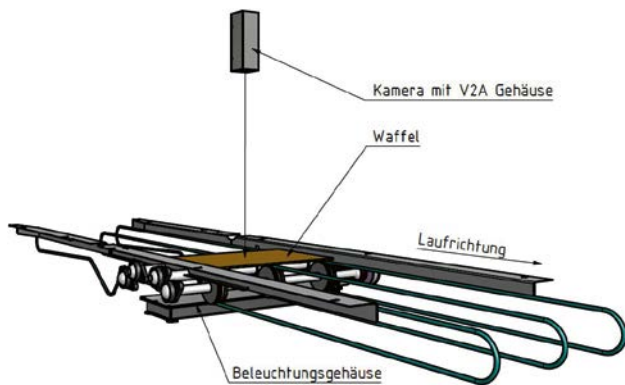
Schematische Darstellung der Systemkomponenten
