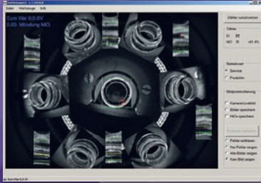
Leerflascheninspektion – Ergebnisbild der Mündungskontrolle
