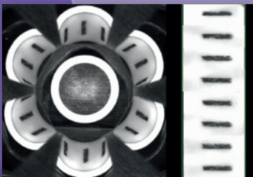
Messung der Zündstrichgeometrie: Kamerabild und Abwicklung mit Zündstrichen
