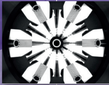
Mantel- und Stirnseitenprüfung von Edelstahlrohren
